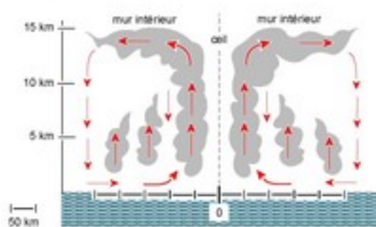
Coupe verticale d'un cyclone tropical
