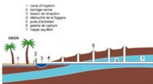
Foggara : schéma de fonctionnement
