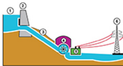
Fonctionnement d'un barrage hydroélectrique
