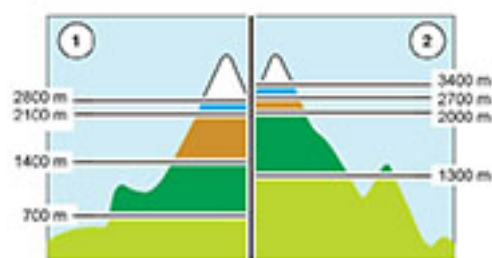
Impact du réchauffement climatique sur l'étagement de la végétation en montagne
