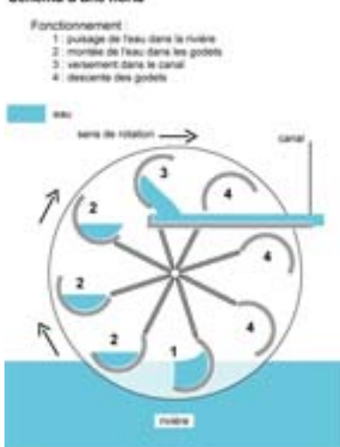
Schéma d'une noria
